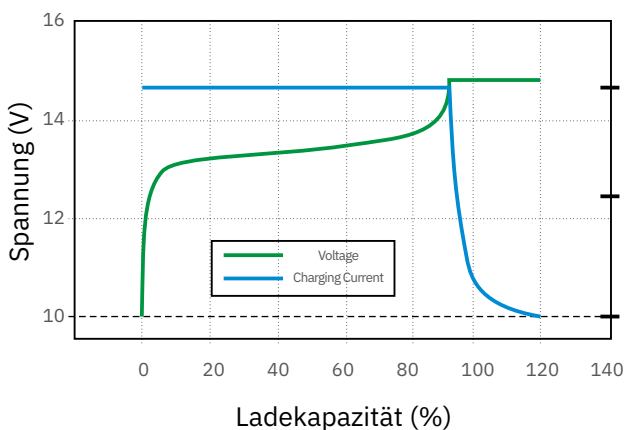
Ladeigenschaften (0,5C bei 20 °C)
